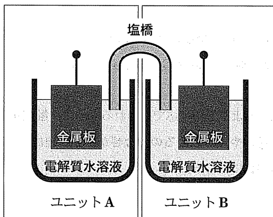
図 ユニットを組み合わせた電池
