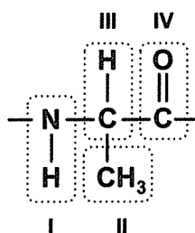
図 タンパク質中のアラニンの構造
